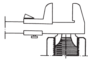
Innendurchmesser
